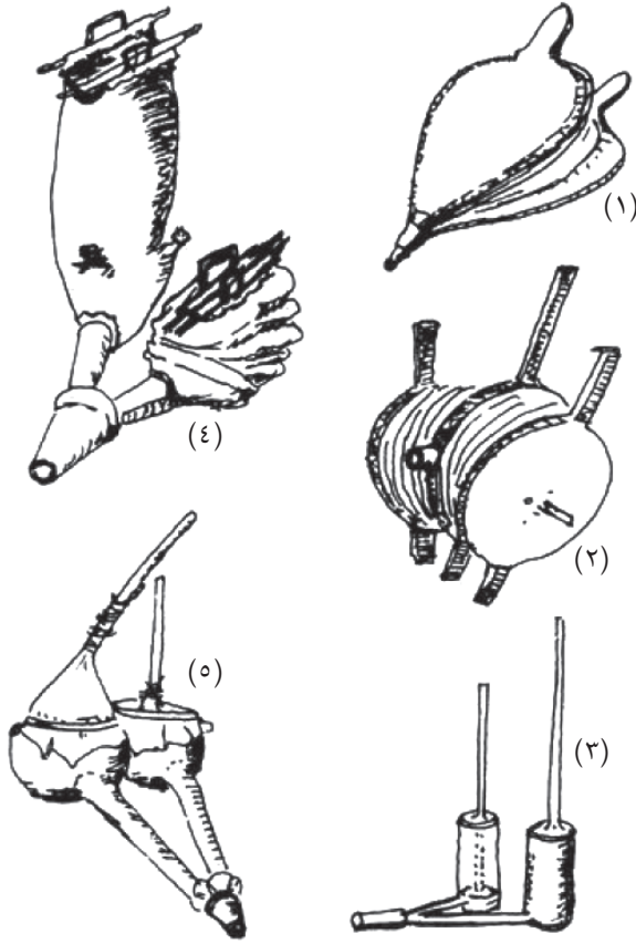
شكل ٦-٢: أنواع الكور البدائية (منفاخ الهواء): (١) و(٢) منفاخ أكورديون. (٣) منفاخ بستون. (٤) و(٥) منفاخ جلدي فخاري.
