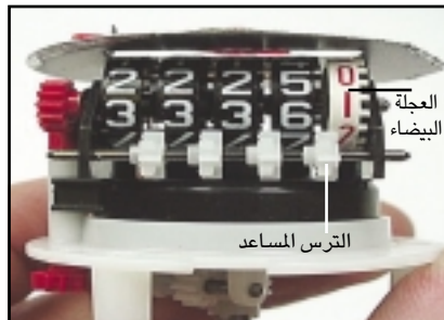
شكل (٣) العجلة البيضاء
