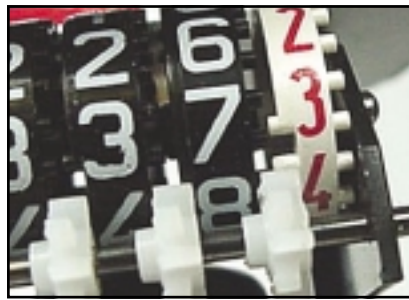
● شكل (٤) الأسفينات الجانبية والتروس المساعدة
