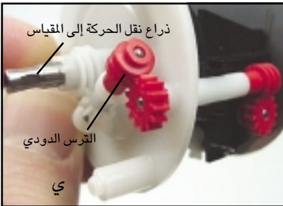
شكل (٢) مجموعات التروس الدودية
