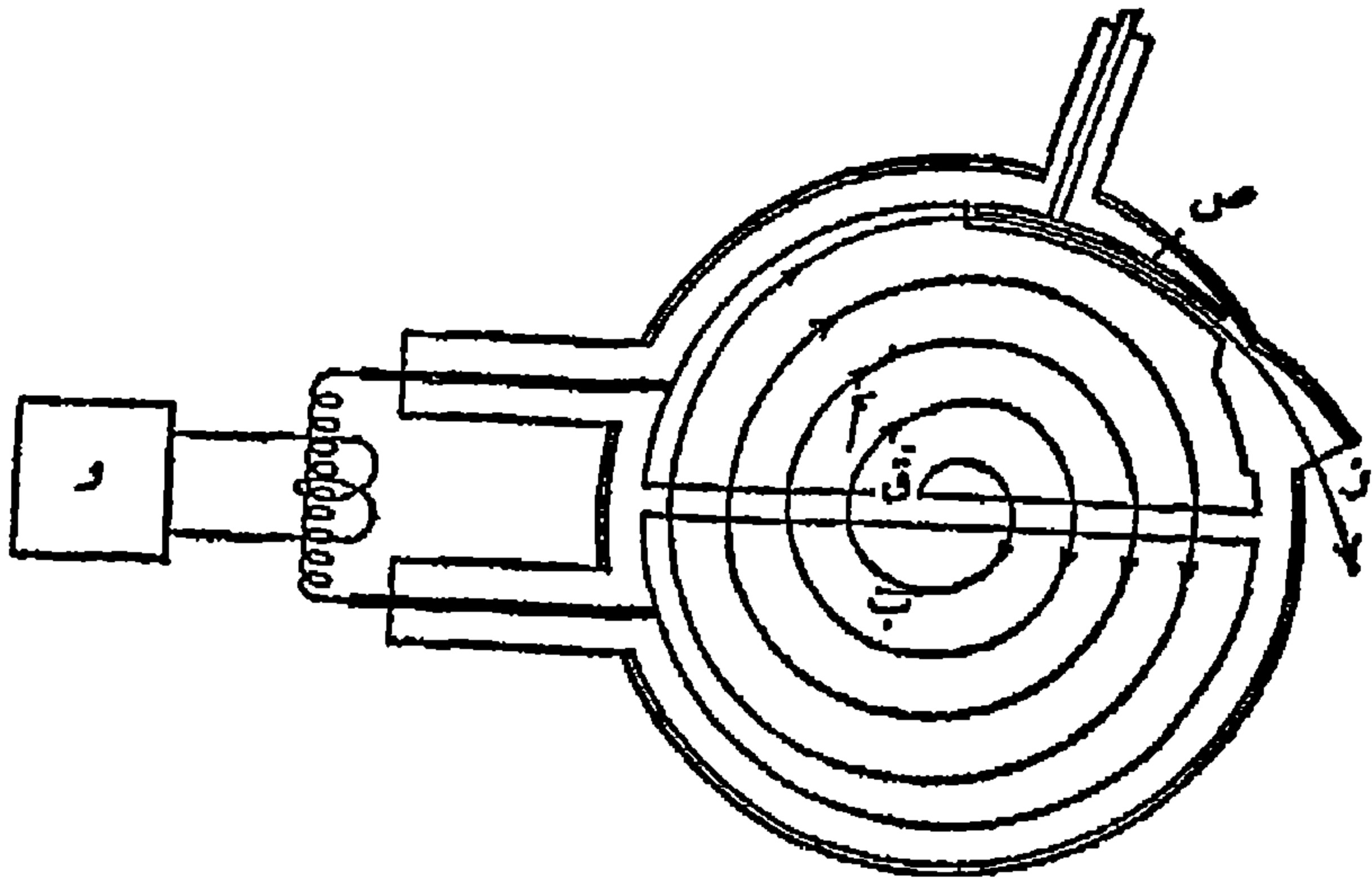
الشكل ٥ . - السيكلوترون
