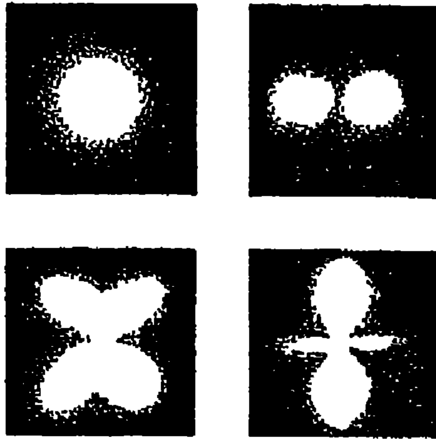
الشكل ٣ . - الذرة حسب الميكانيكا التمرجية
