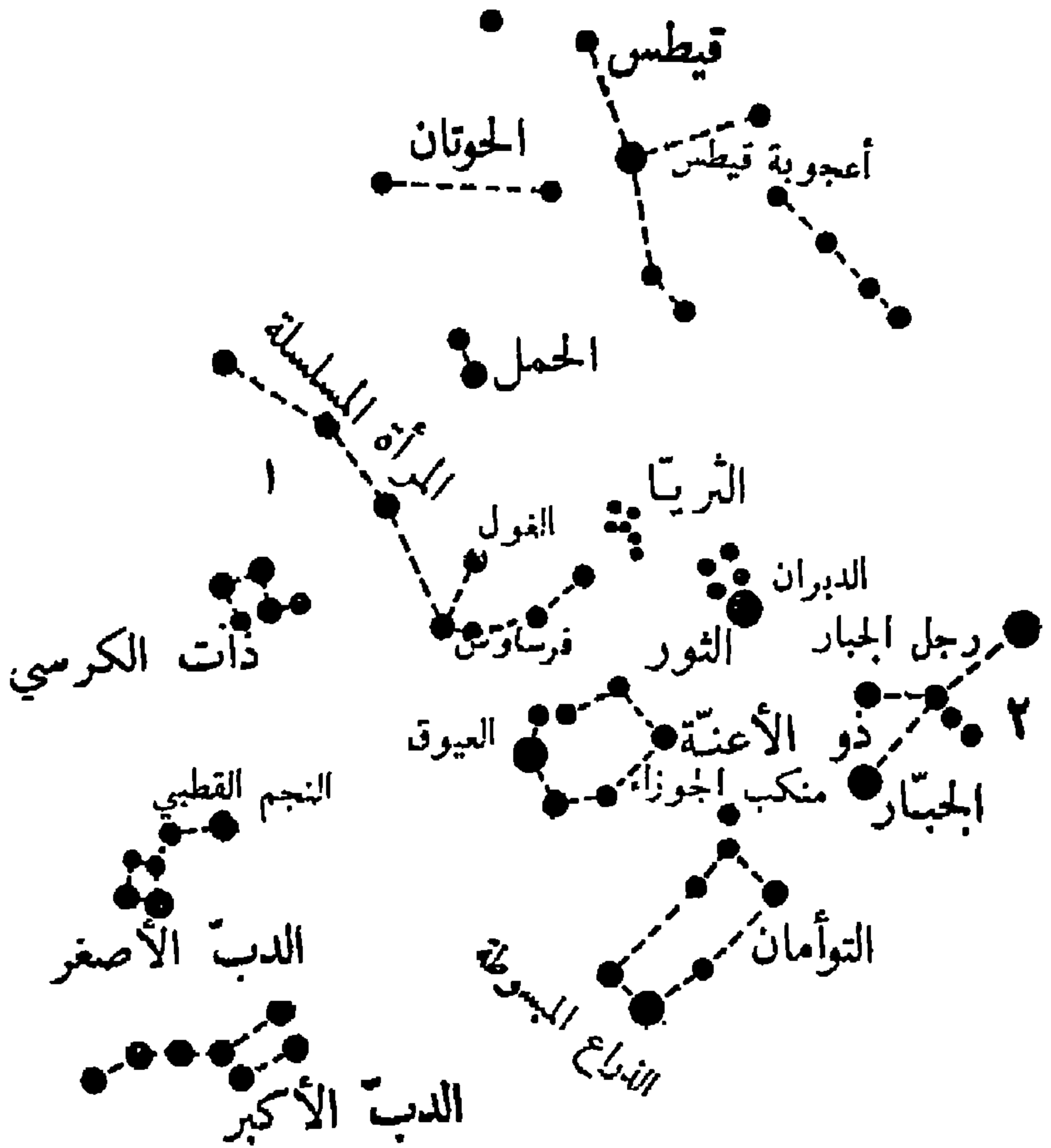
الشكل ٧ . - موقع مجرّة المرأة المسلسلة (١+) وسديم الجبار (٢) في السماء الشمالية
