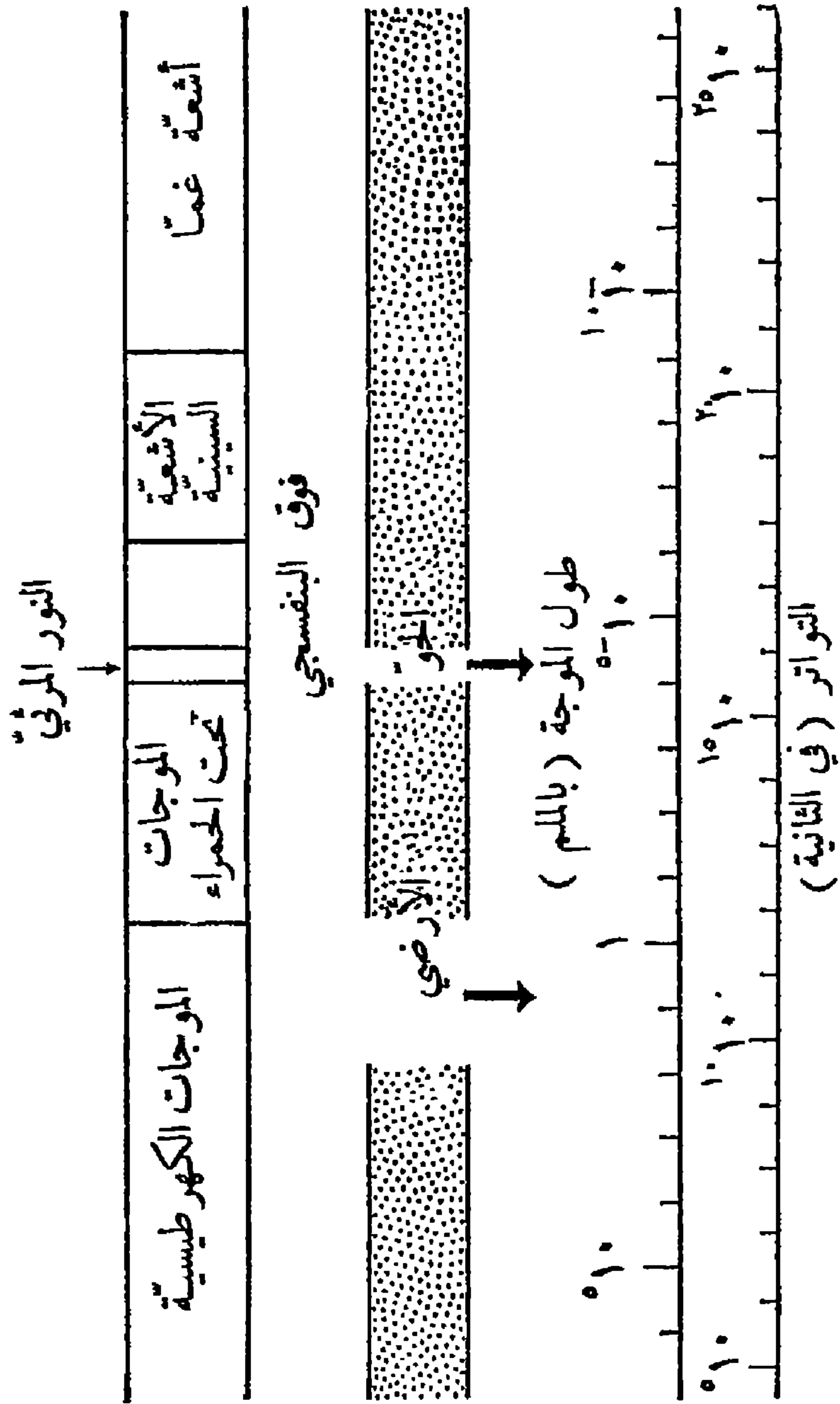
شكل ٦ - لا تستطيع الإشعاعات الكهروطيسية المختلفة اختراق جونا إلا من كوتين . يظهر في أسفل الشكل تواتر هذه هذه الإشعاعات وأطوال موجاتها .
