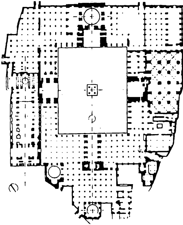
شكل (٢٧): مسجدي جامع بأصفهان (عن جروبه).
