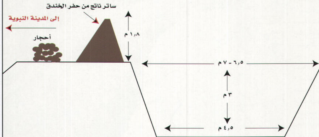
الأبعاد التقريبية للخندق
