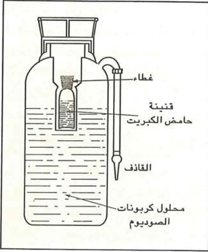
● شكل (٣) مكونات مطفأة الصودا والحامض .
