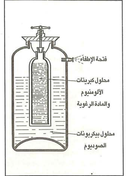
• شكل (٤) مكونات المطفاة اليدوية للسائل الرغوي .
