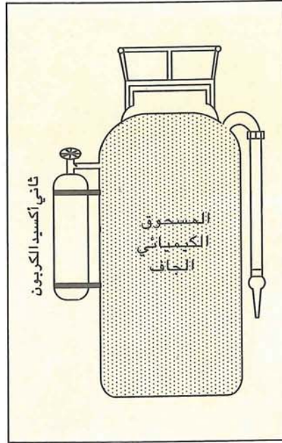
• شكل (٥) مكونات مطفاة المسحوق الكيميائي الجاف .
