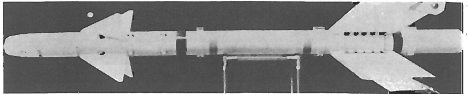
صورة رقم 31 : صاروخ جو جو Python 3 (إسرائيلي) .
