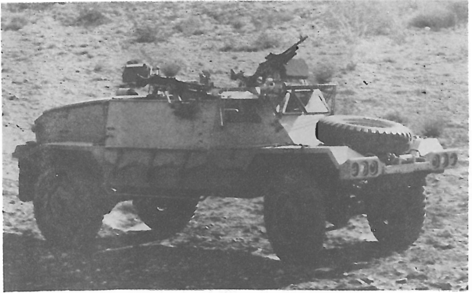
صورة رقم 42 : عربة مدرعة RAM-VI (إسرائيلي) .
