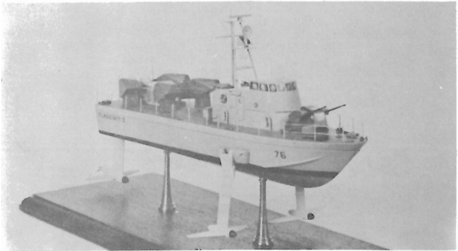
صورة رقم 58 : هيد روفيل Flagstaff II (صناعة أمريكية) . إسرائيل حصلت على حق تصنيعه النموذج الذي في الصورة يحمل 4 صاروخ جابريل (إسرائيلي) + 1 مدفع 30 ملم ثنائي + 1 مدفع 20 ملم ثنائي .
