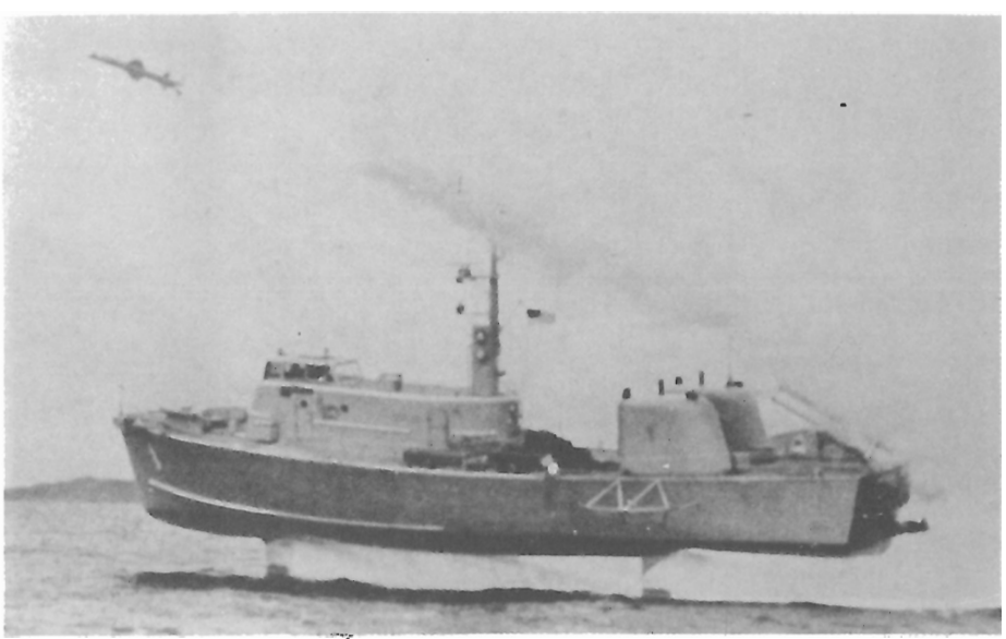
صورة رقم 57 : هيد روفيل PCH-1 High Point (صناعة أمريكية) . تحمل 2 صاروخ Harpoon الحمولة العادية 110 طن ، وأقصى حمولة 131 طن (الحمولة المفيدة 27.6 طن) . السرعة 50 عقدة .
