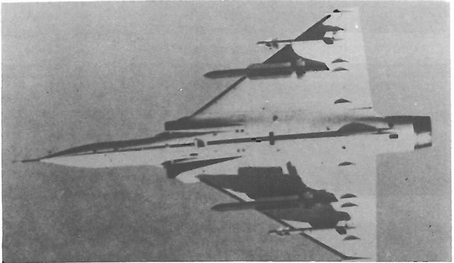
صورة رقم 30 : صواريخ جو جو مثبتة في بطن الطائرة ميراج 2000 . من الداخل 2 Super 530 ، من الخارج 2 R 550 Magic
