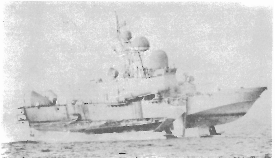
صورة رقم 56 : هيدروفيل Sarancha (صناعة سوفيتية) تحمل 4 صاروخ SS-N-9 + قاعدة صواريخ سطح جو ومعها 15 - 20 صاروخ + مدفع 30 ملم . السرعة 50 عقدة أقصى حمولة 330 طن .
