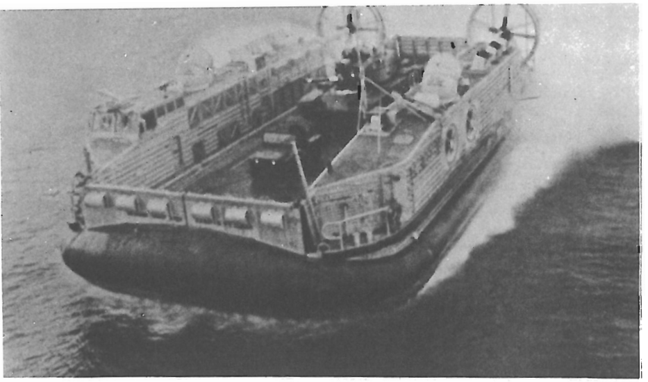
صورة رقم 55 : مركبة وسادة هوائية jeff-B (صناعة أمريكية) . تستطيع حمل 1 دبابة + 1 عربة مدرعة باجمالي 54 413 كجم ، السرعة 50 عقدة ، والمدى 200 ميل ، أقصى حمولة 165 طن .
