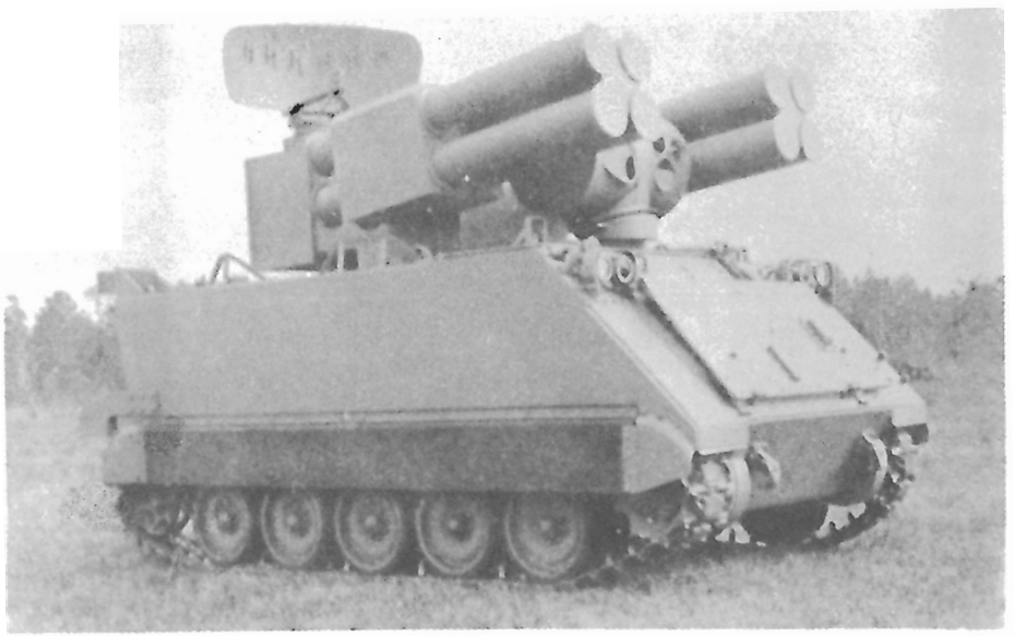
صورة رقم 4 : صاروخ ADATS (دولي) فوق مركبة M-113 ويستخدم ضد الطائرات ، ضد الدبابات .
