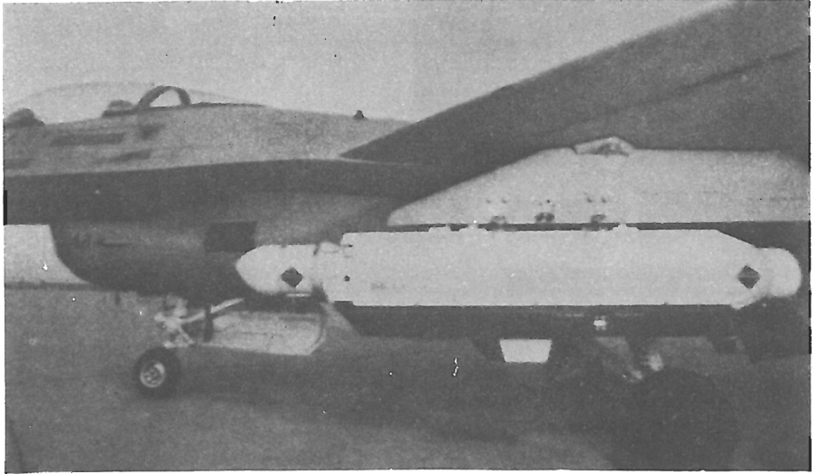
صورة رقم 40 : مستودع الاجراءات الالكترونية المضادة ALQ-131 (أمريكي) . مثبت تحت جناح الطائرة F-16
