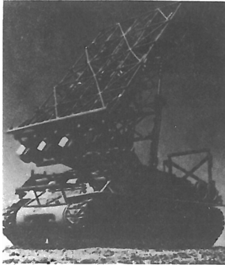
صورة رقم 46 : راجمة صواريخ 290 ملم (إسرائيلي) .
