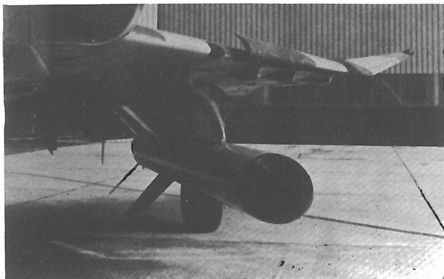
صورة رقم 26 : صاروخ جو سطح Gabriel (إسرائيلي) مثبت أسفل جناح طائرة F-4
