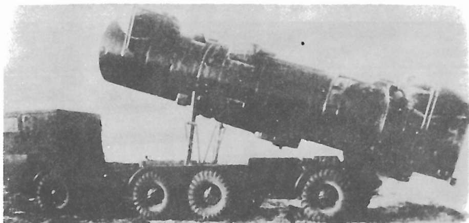
صورة رقم 10 : صاروخ Sepal SSC-1B للدفاع الساحلي (سوفيتي) .
