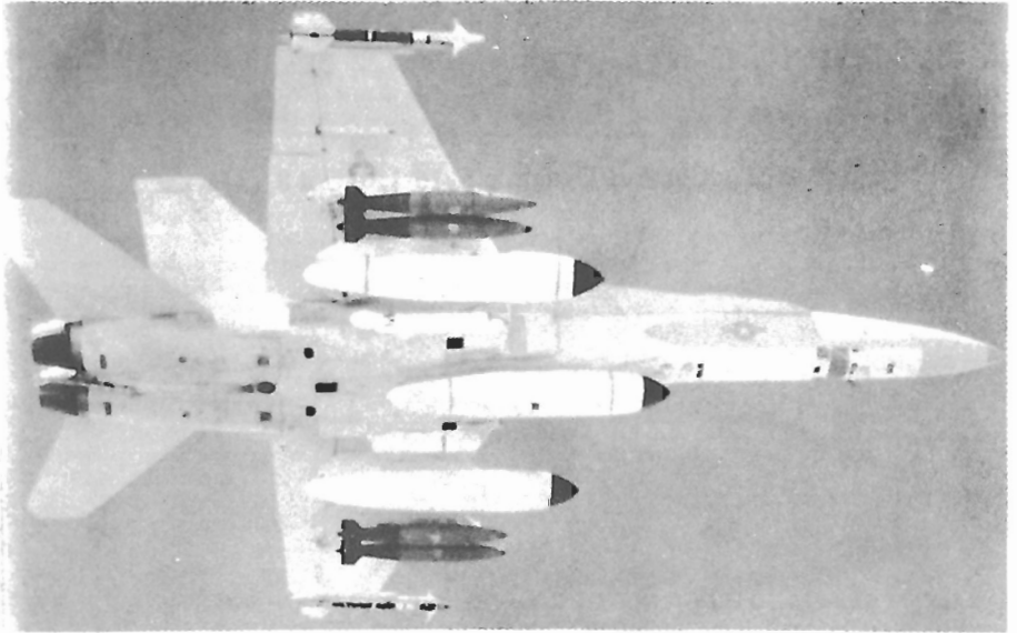
صورة رقم 51 . Mac Donald Douglas F/A 18 A Hornet تحمل أسلحة من الخارج للداخل ما يلي (2 صاروخ Sidewinder ، 4 قنبلة كل منها 1000 رطل ، 3 مستودع وقود احتياطي) وبين مستودعات الوقود الاحتياطي يوجد أسطوانة خاصة بالاعاقة الالكترونية المضادة ، أسطوانة خاصة باكتشاف الليزر . (صناعة أمريكية) :
