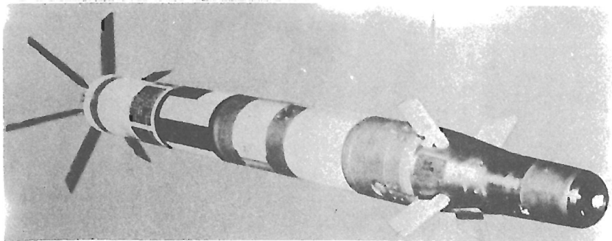
صورة رقم 14 : قذيفة مدفع عيار 5 بوصة (أمريكي) مجهزة برأس باحث عن الليزر.
