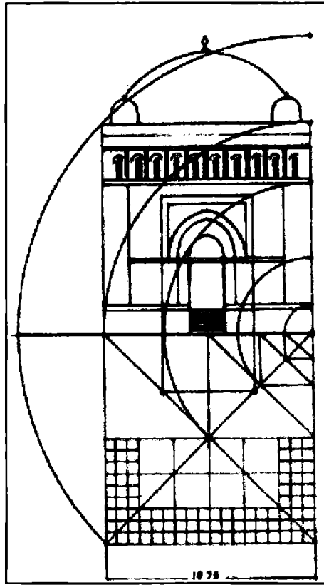
شكل (٣٦): نموذج لواجهة مثمنة مصممة طبقاً لنسب هندسية محددة.
